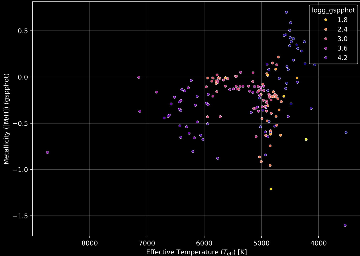
APOGEE DR17 Field: [280+49] Stellar Population Parameters (n= 173)
